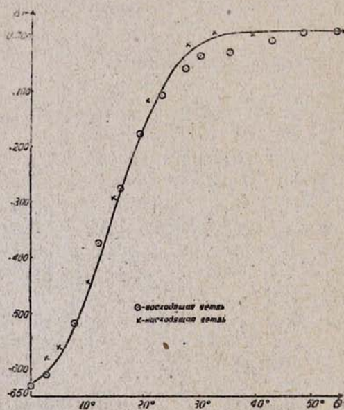
Отраженная теоретическая кривая блеска CG Cygni
